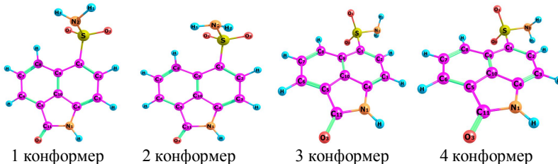
Рис. Геометрическое строение конформеров C_{11}H_8SO_3N_2
